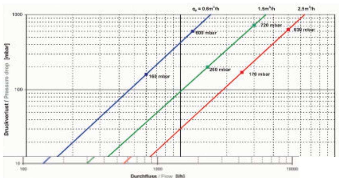
Druckverlustdarstellung des Einstahl-Kompaktwärmezählers "Calidus-tec"
