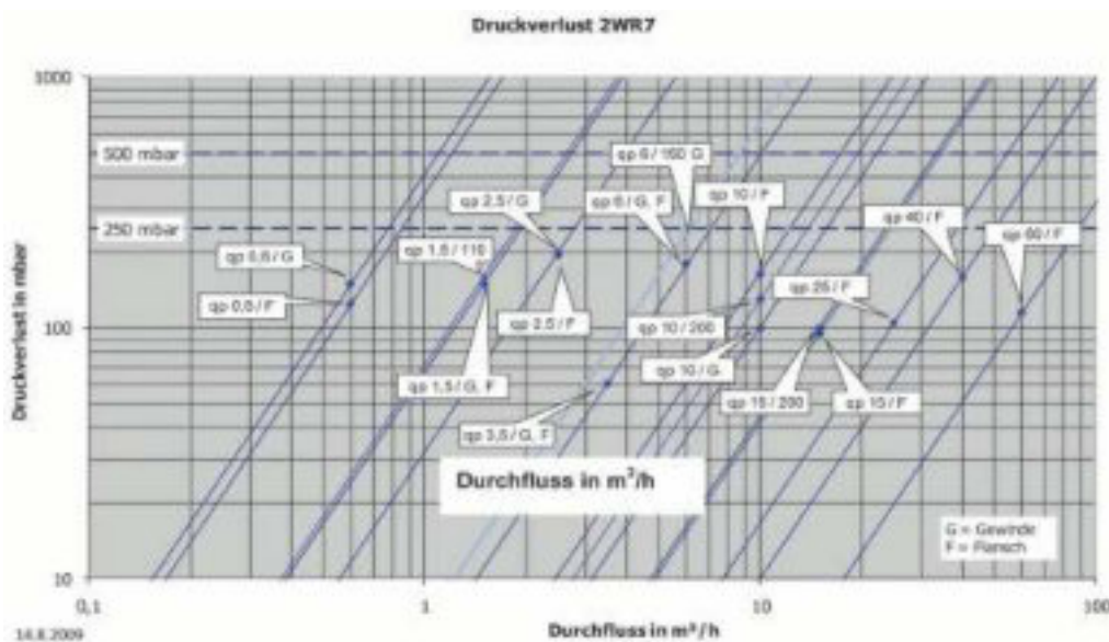
Druckverlustdarstellung des Ultraschallzählers "Calidus-tec"
