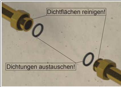
Montageschritt 3
