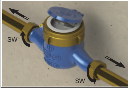
Montageschritt 1
