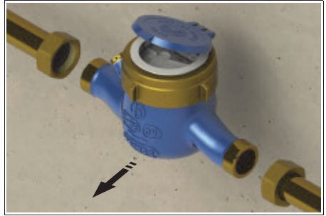
Montageschritt 2
