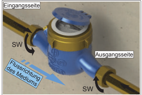
Montageschritt 4
