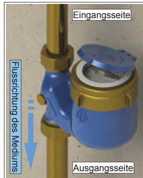
Einbau Fallrohr
