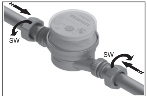
Montageschritt 4
