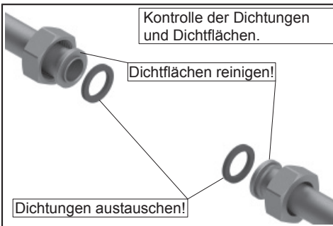
Montageschritt 3
