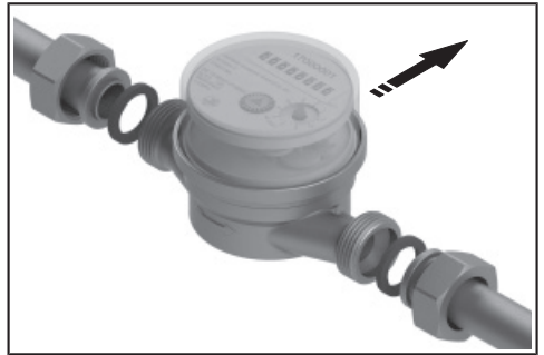
Montageschritt 2
