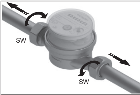
Montageschritt 1
