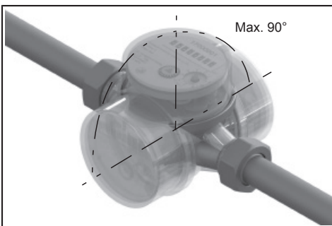
Montageschritt 5
