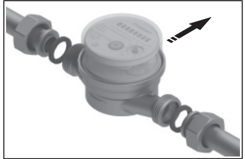
Montageschritt 2
