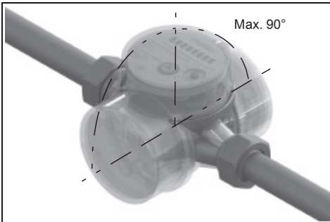
Montageschritt 5
