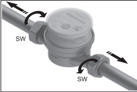
Montageschritt 1
