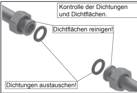
Montageschritt 3
